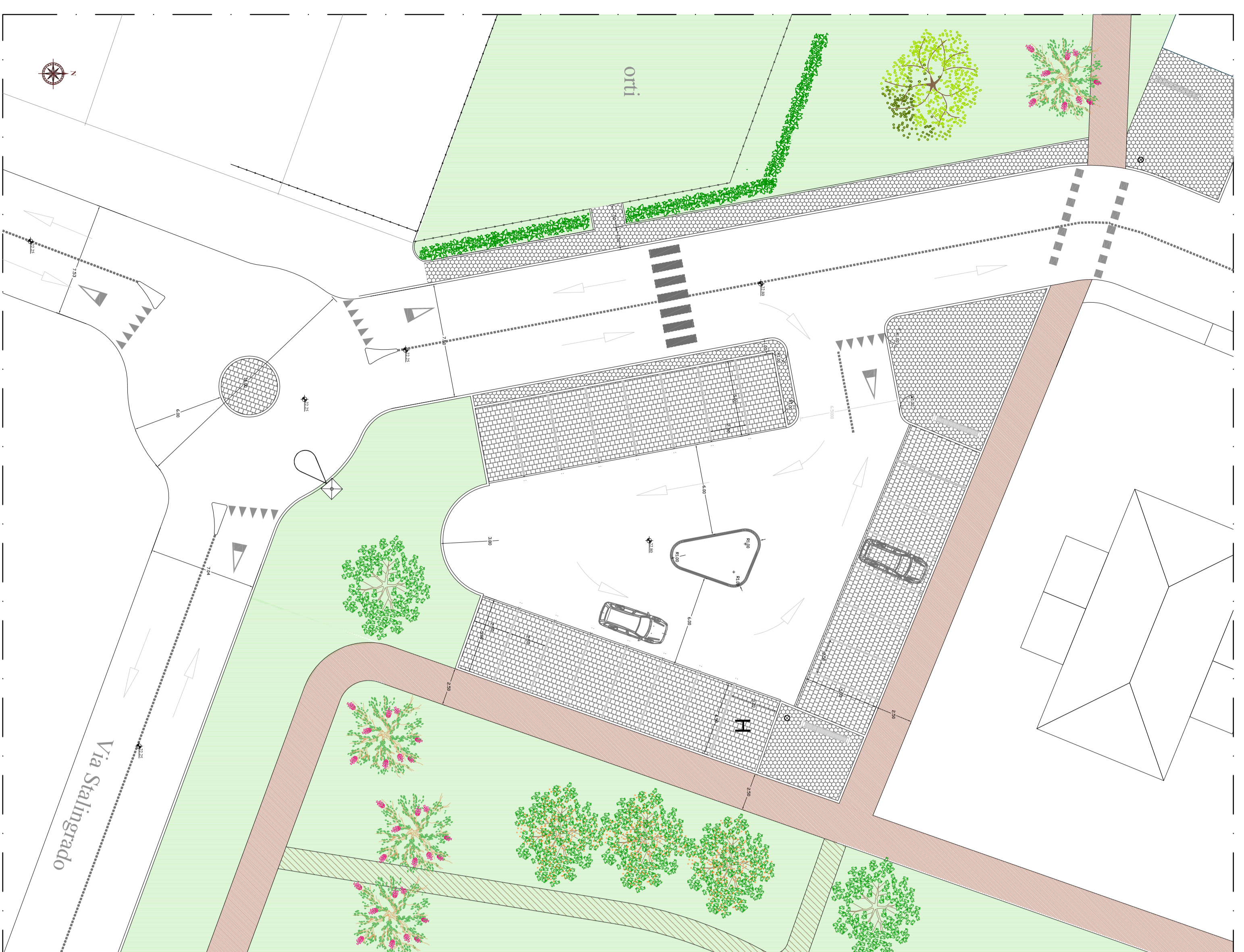
PIANTA PARCHEGGI INGRESSO COMPARTO SCALA 1:200
